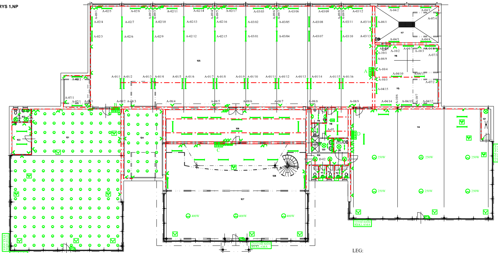
TABULKA MÍSTNOSTÍ 1NP
